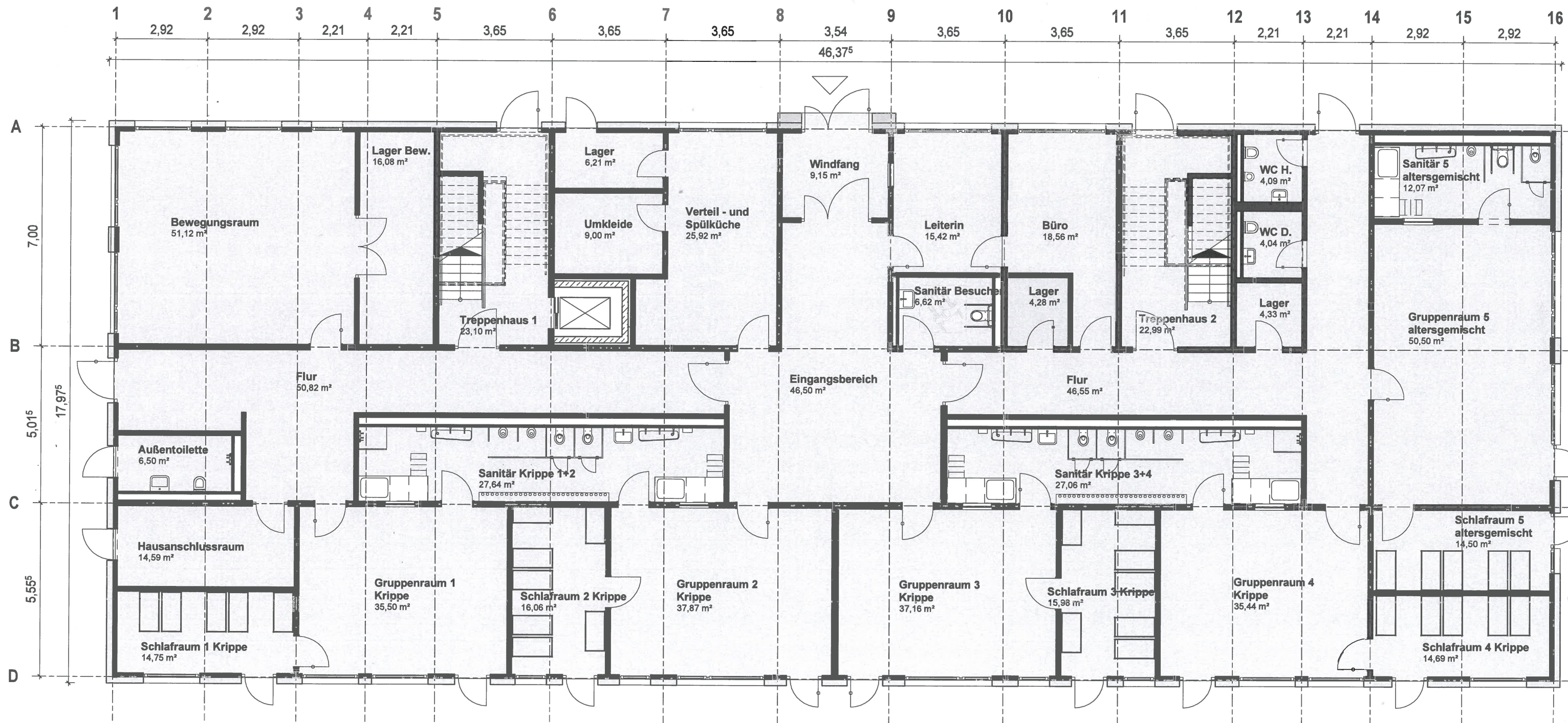
Beispiel Grundriss EG
